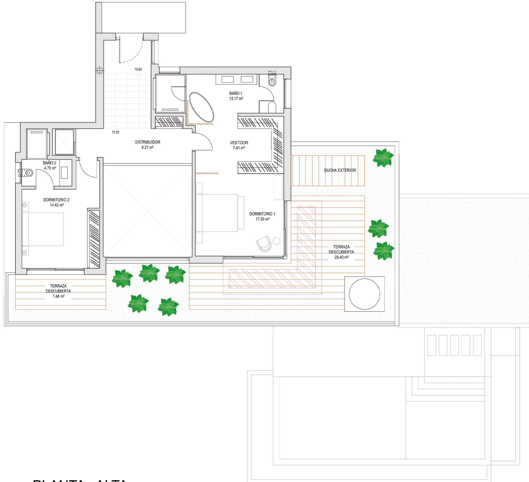
PLANTA ALTA
