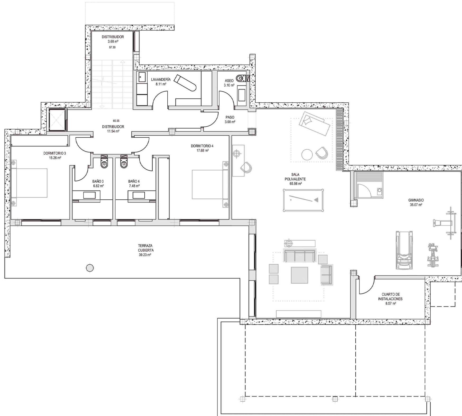
PLANTA SOTANO
